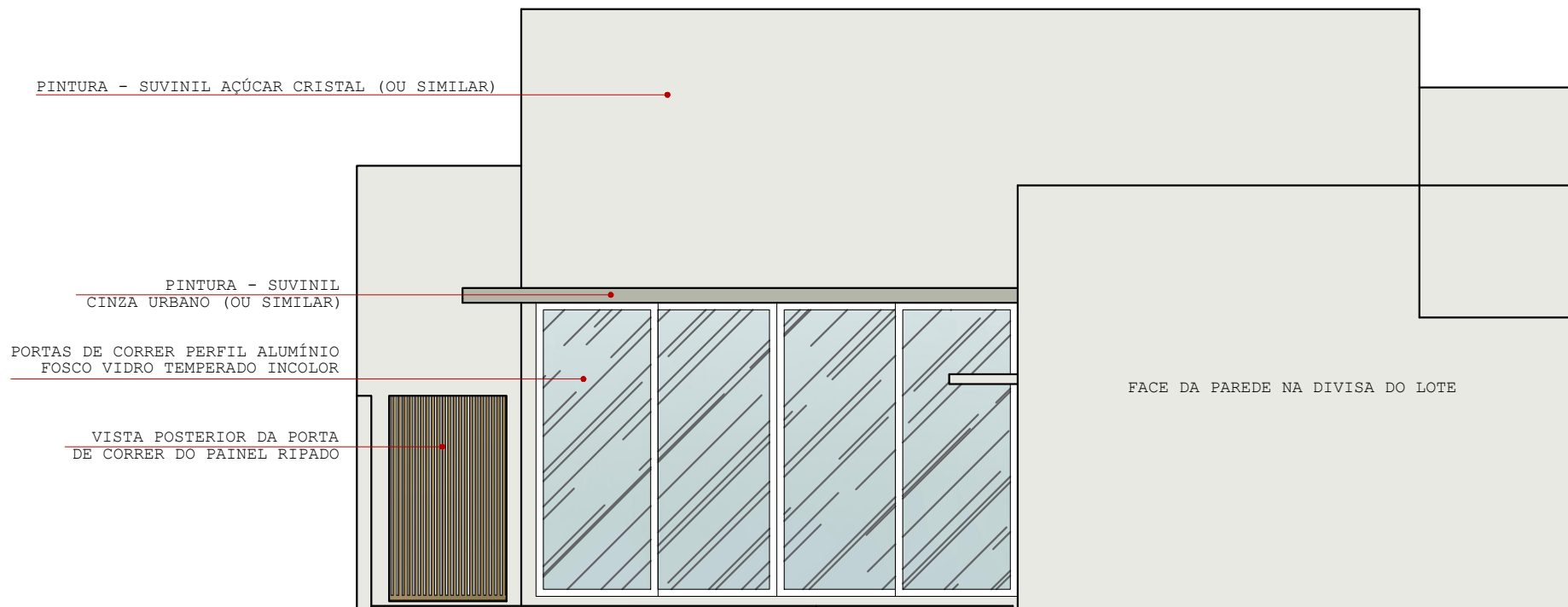
4 FACHADA POSTERIOR ESC.: 1/75
