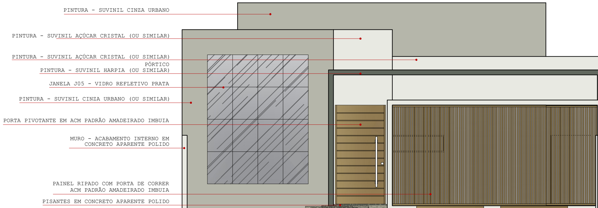
3 FACHADA FRONTAL ESC.: 1/75
